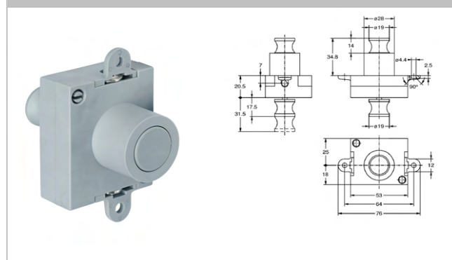
8628 Drehstangenschloss
