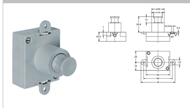
8618 Drehstangenschloss
