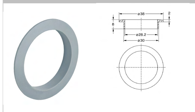
7433 Rosette rund
