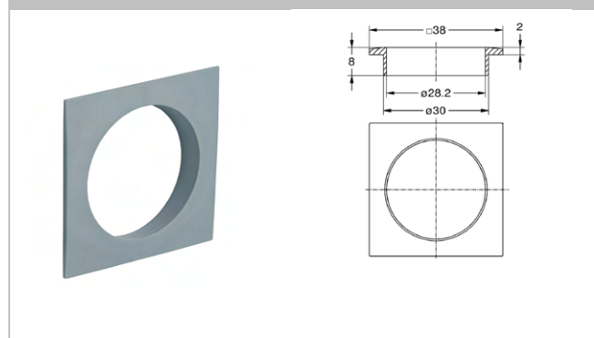
7432 Rosette eckig
